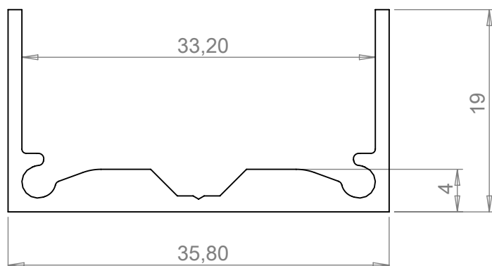
Montant de côté 60372X 410,64 g/m
