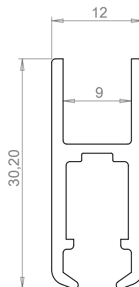
Sabot 60369U 325,62 g/m
