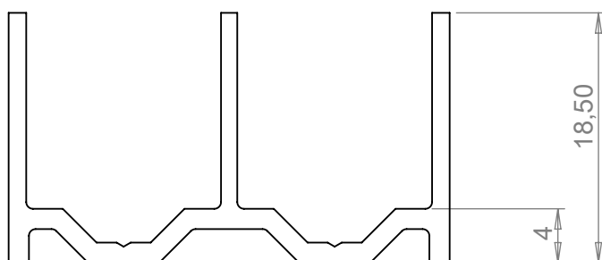
Coulisse haute 60366R 317,9 g/m
